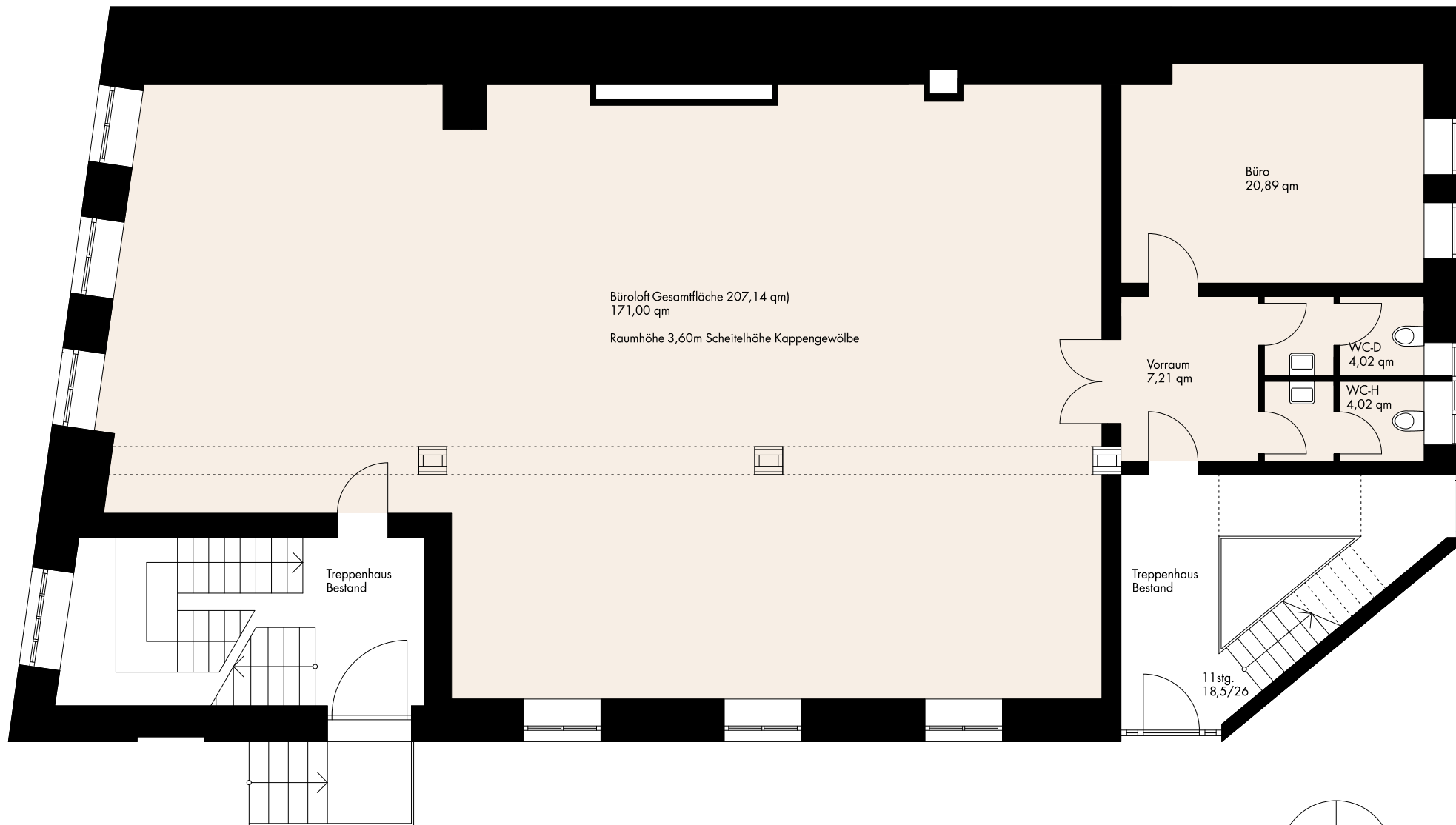
Wohnhaus Kirchenstr. 15 Grundriss EG M 1:100 Gestaltungsvariante II - Bestand Büronutzung
