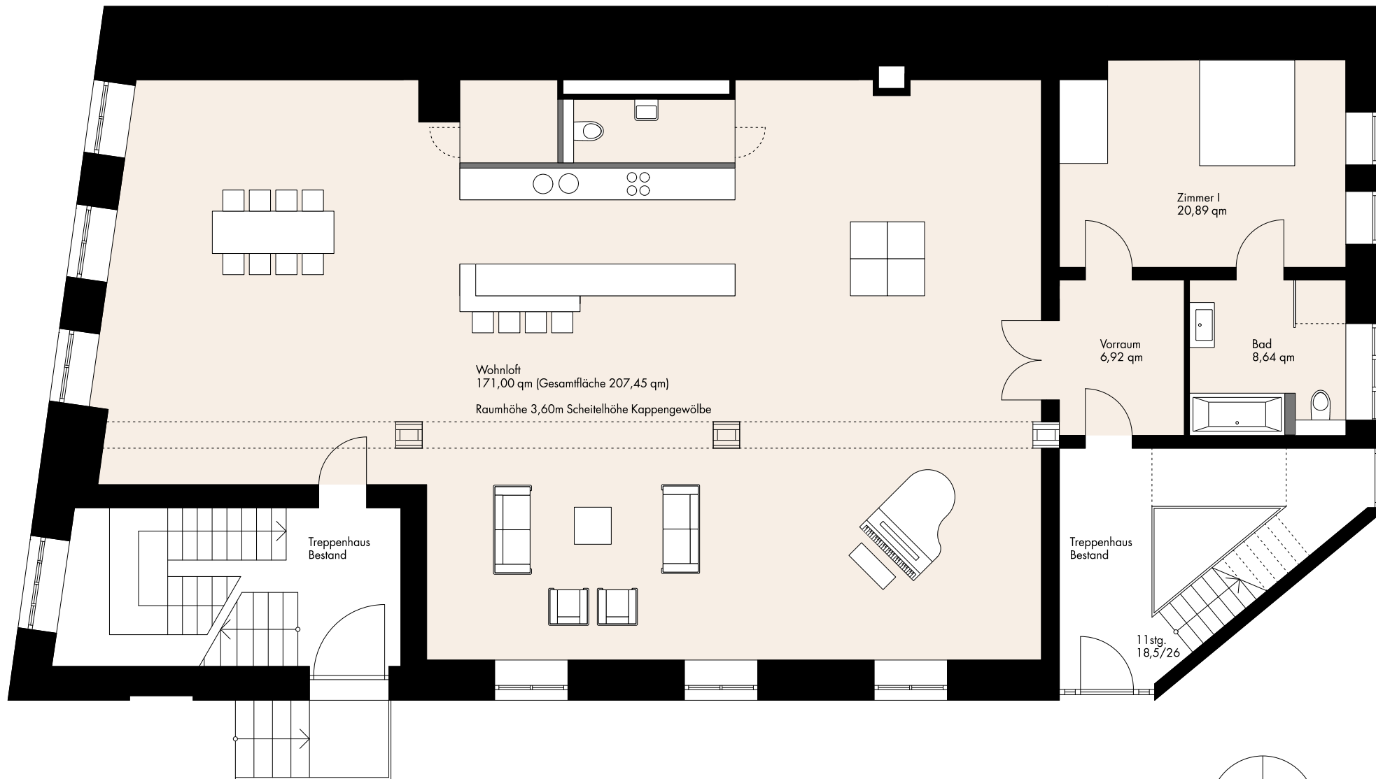
Wohnhaus Kirchenstr. 15 Grundriss EG M 1:100 Gestaltungsvariante (individueller Ausbau möglich)
